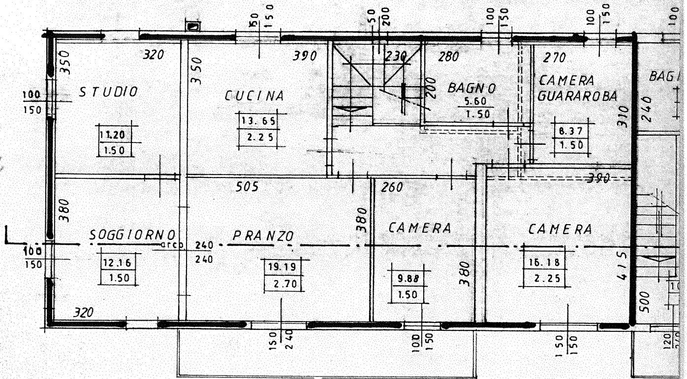
PIANO PRIMO
