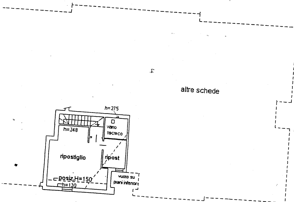
PIANTA PIANO SECONDO ALTEZZA DI PIANO CM. 270
