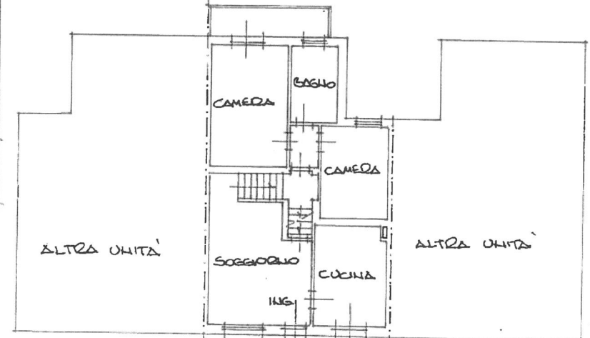
PIANO TERRA E PRIMO H=270
