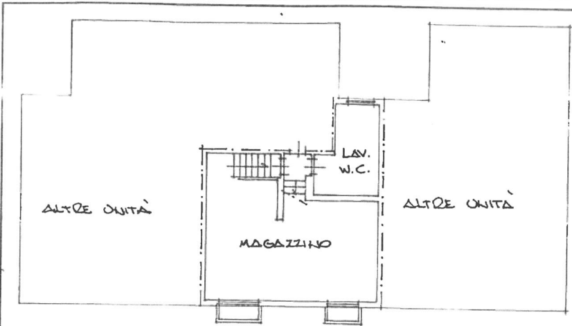
PIANO SEMINTERATO E TERRA H=210
