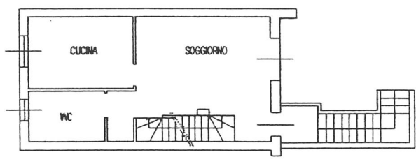
PIANTA PIANO PRIMO H= 2.70
