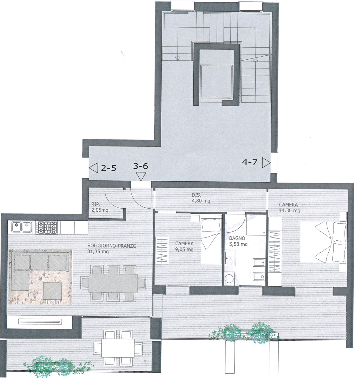
PLANIMETRIA APPARTAMENTO 03_06 - SCALA 1:100
